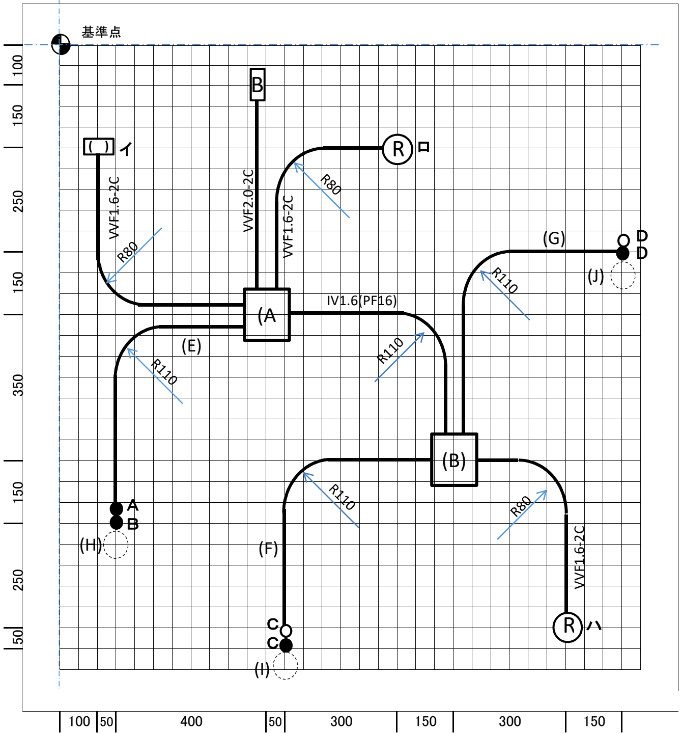
分電盤配置図
