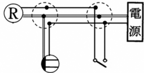
複線図
