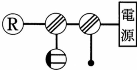
単線図
